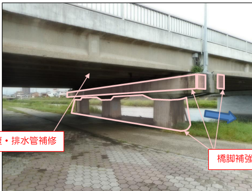
右岸側（南側）橋脚
